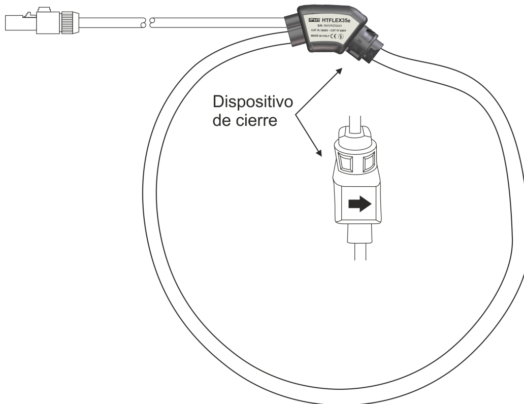
Fig. 2: Descripción de transductor HTFLEX35e
